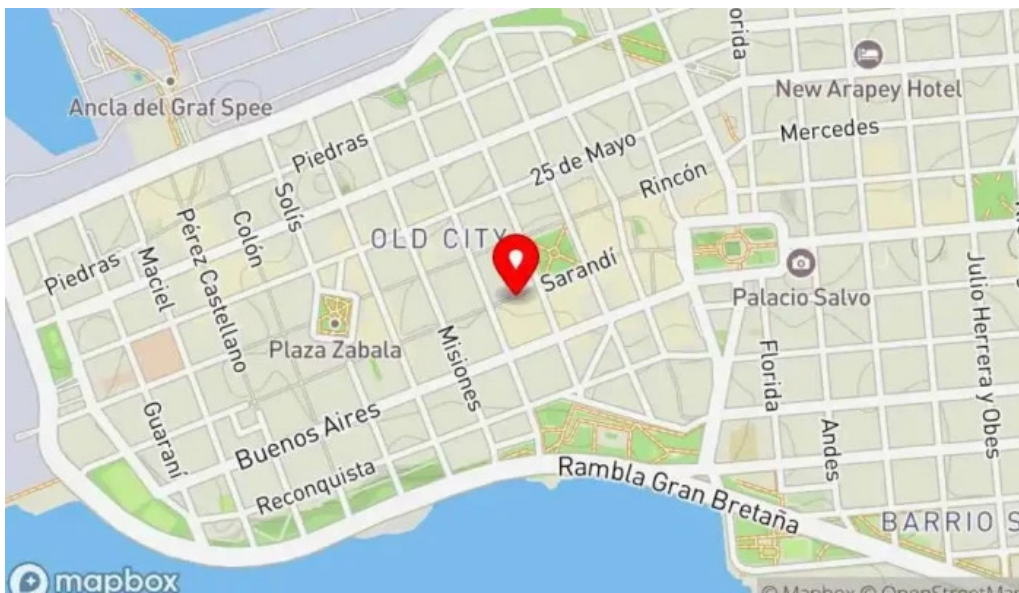
Sinestesia mapa
